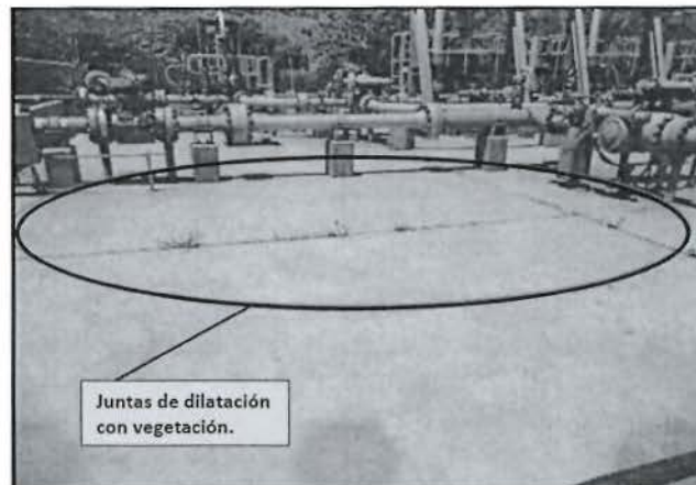
Fotografía N° 4: En las pozas de contingencia de las estaciones de válvulas no presentan adecuada impermeabilización de las juntas de dilatación.
